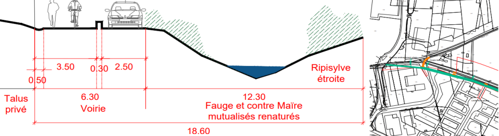
Section C-D
