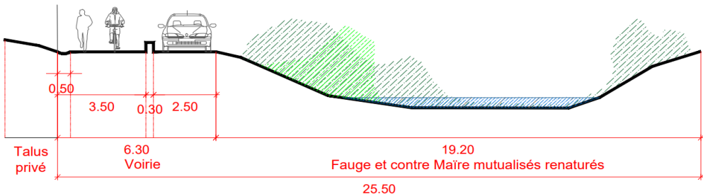
Section C-D
